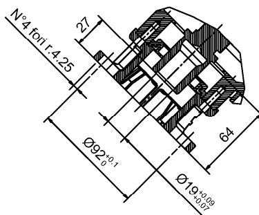
Sez. G-G
